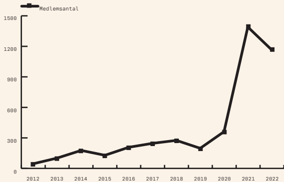
MEDLEMSANTAL
