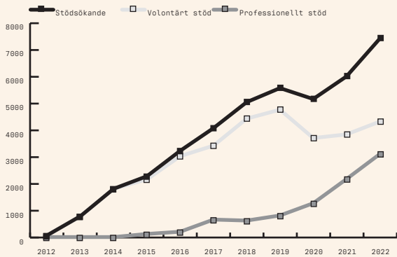
ÅRSARBETSKRAFT
